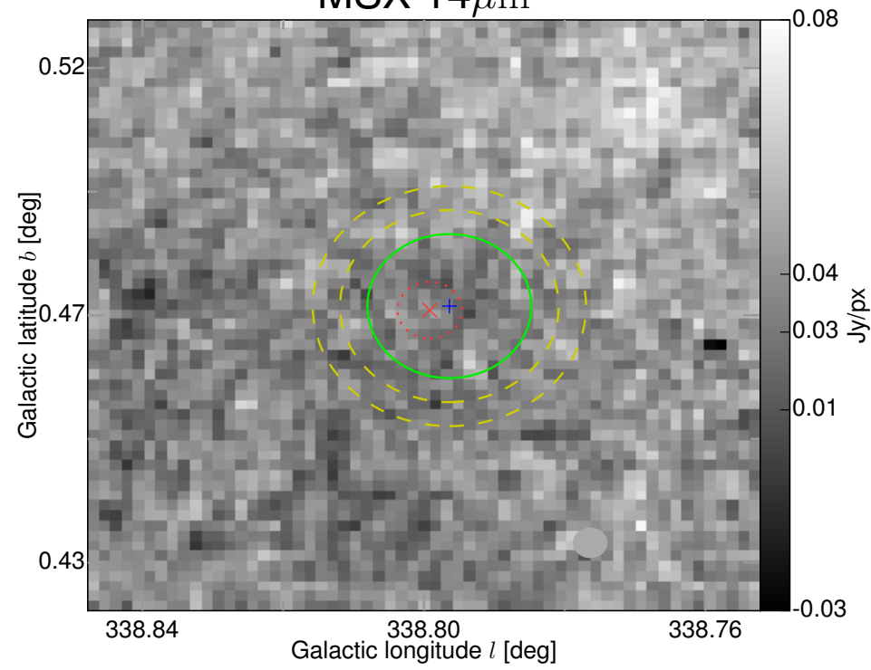
MSX 14 \mu\text{m}
