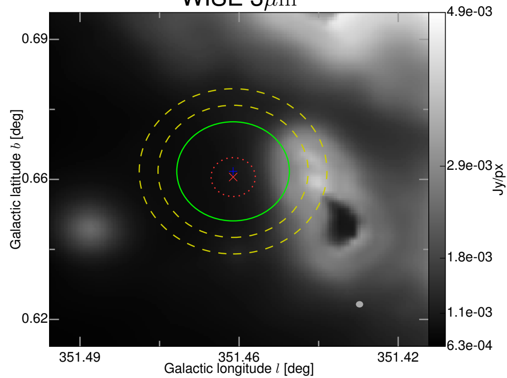
WISE 3\mu\text{m}
