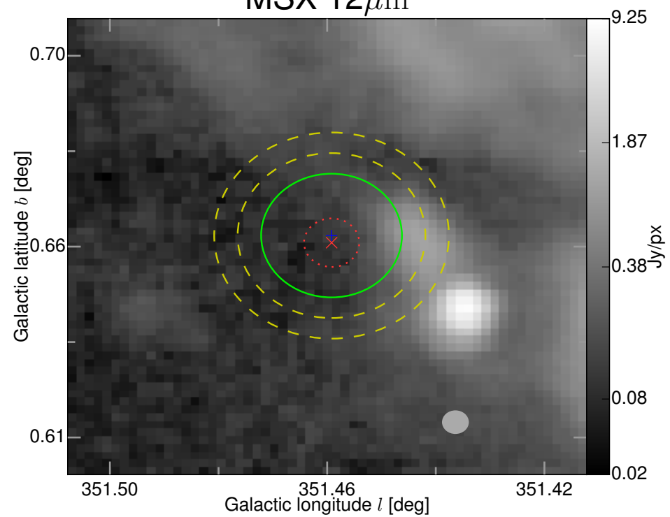
MSX 12\mu\text{m}
