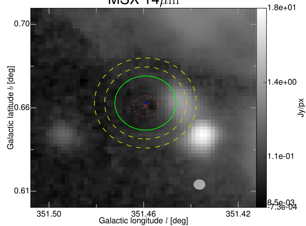
MSX 14\mu\text{m}
