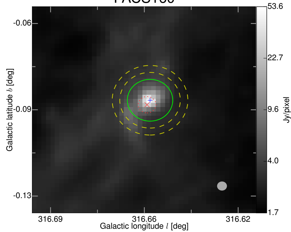
PACS160
