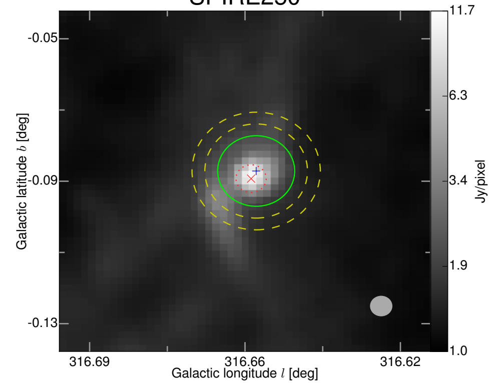
SPIRE250
