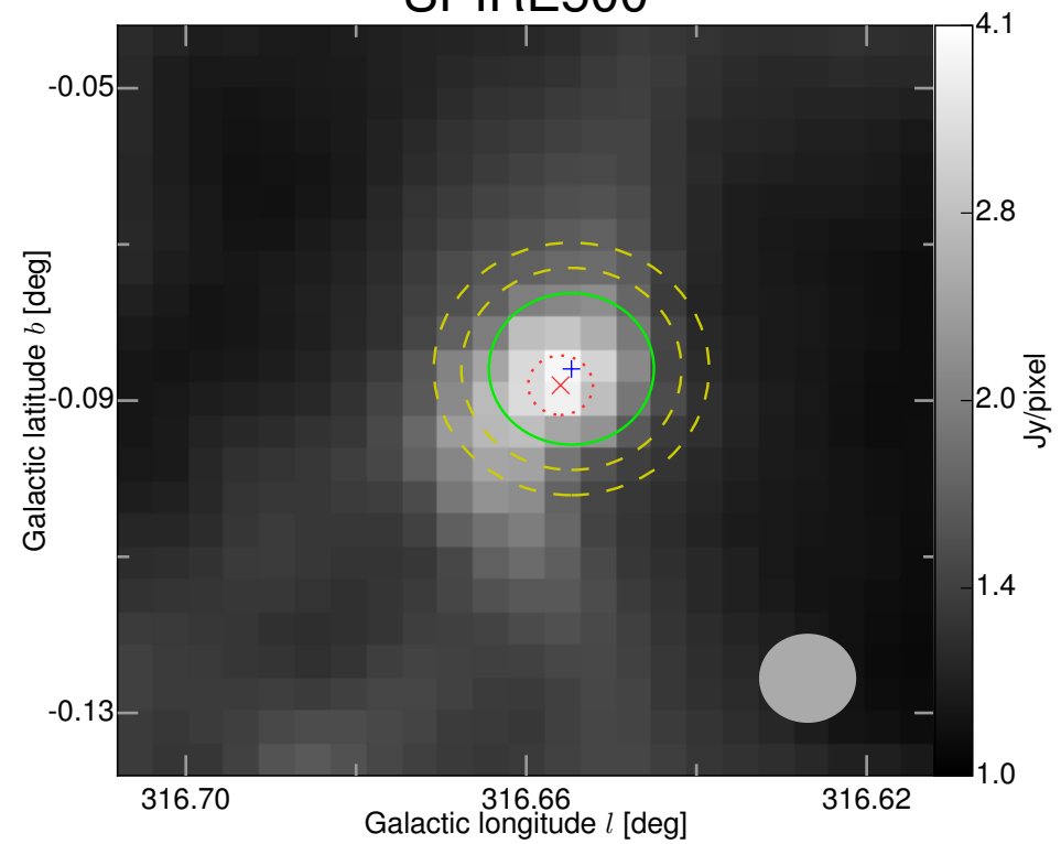
SPIRE500
