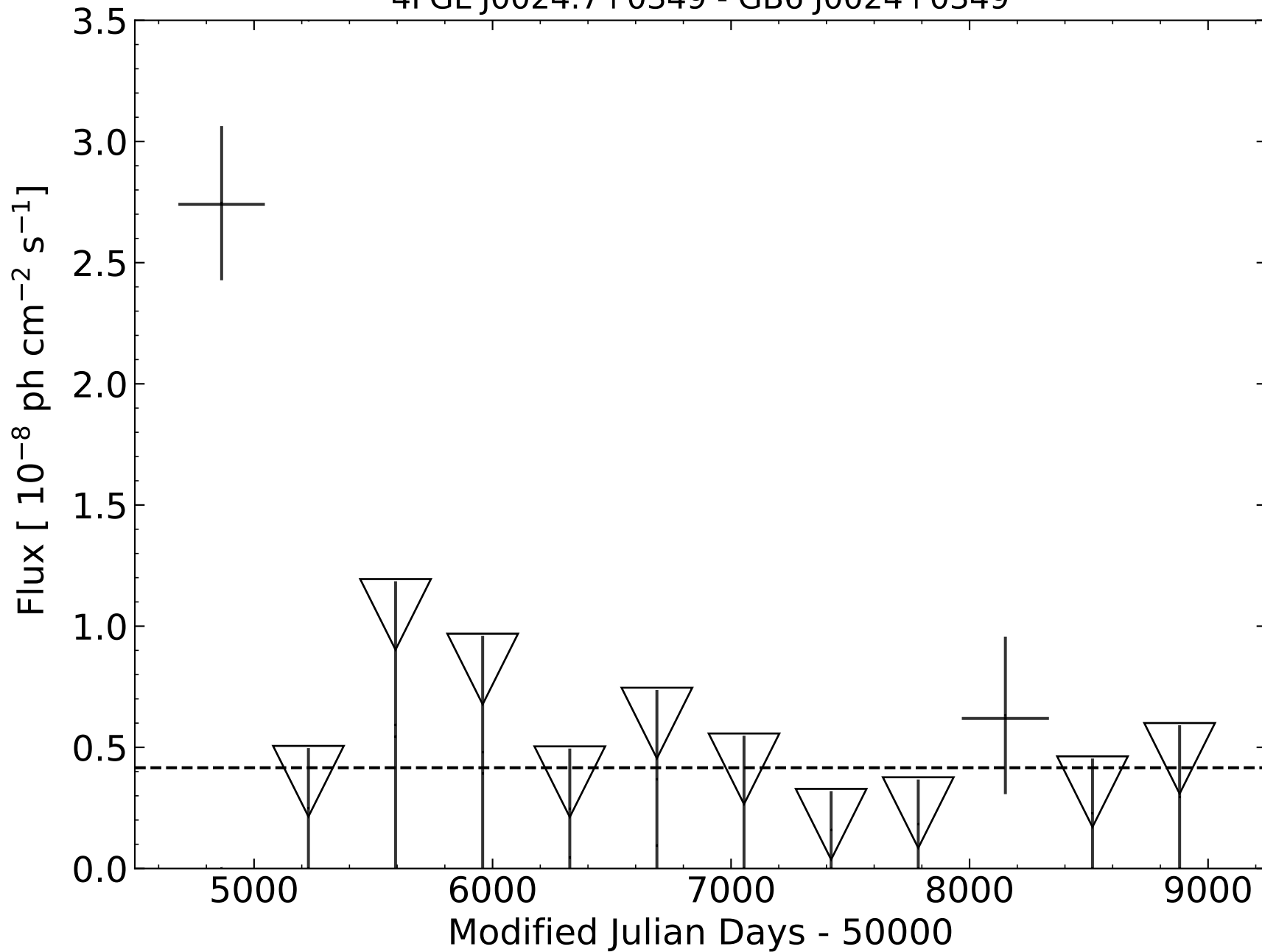
4FGL J0024.7+0349 - GB6 J0024+0349
