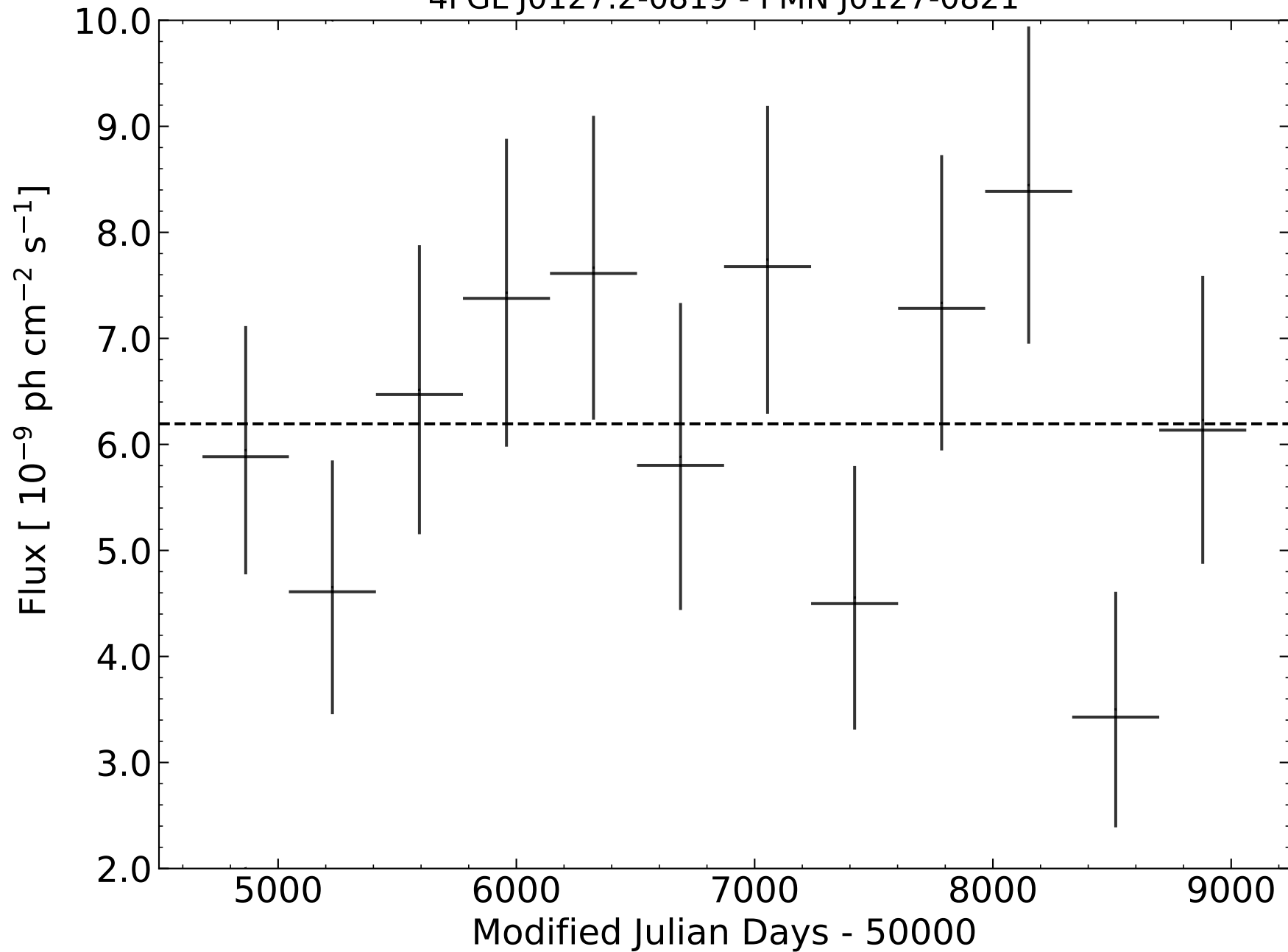
4FGL J0127.2-0819 - PMN J0127-0821
