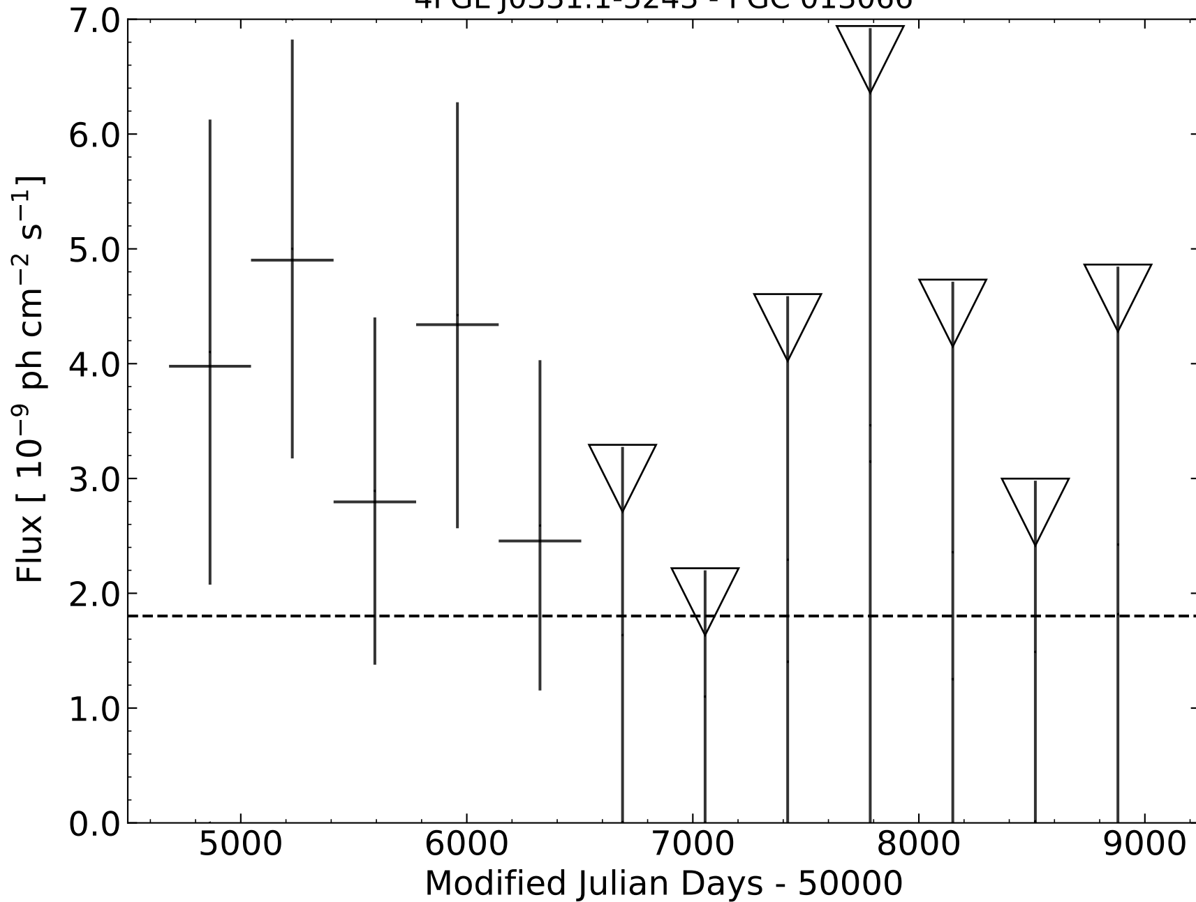
4FGL J0331.1-5243 - PGC 013066
