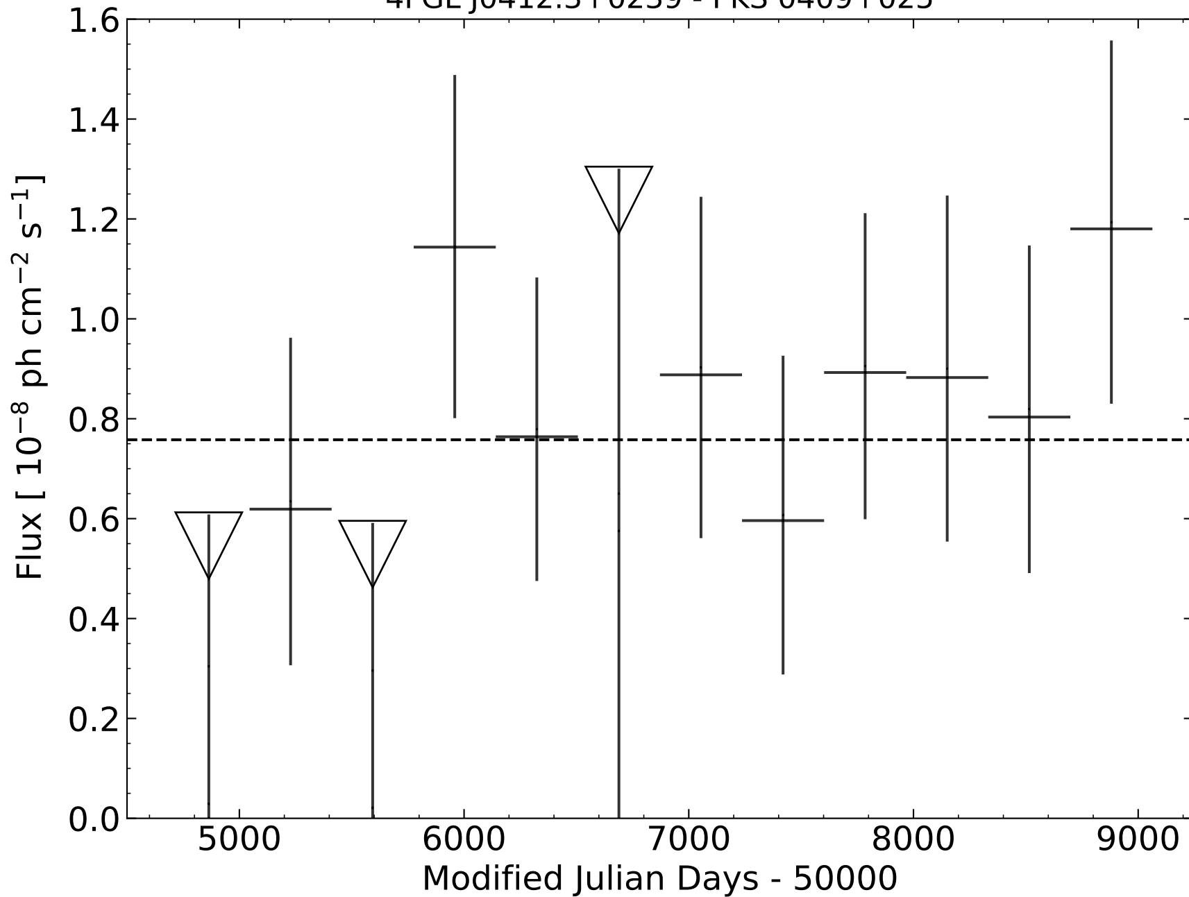
4FGL J0412.3+0239 - PKS 0409+025
