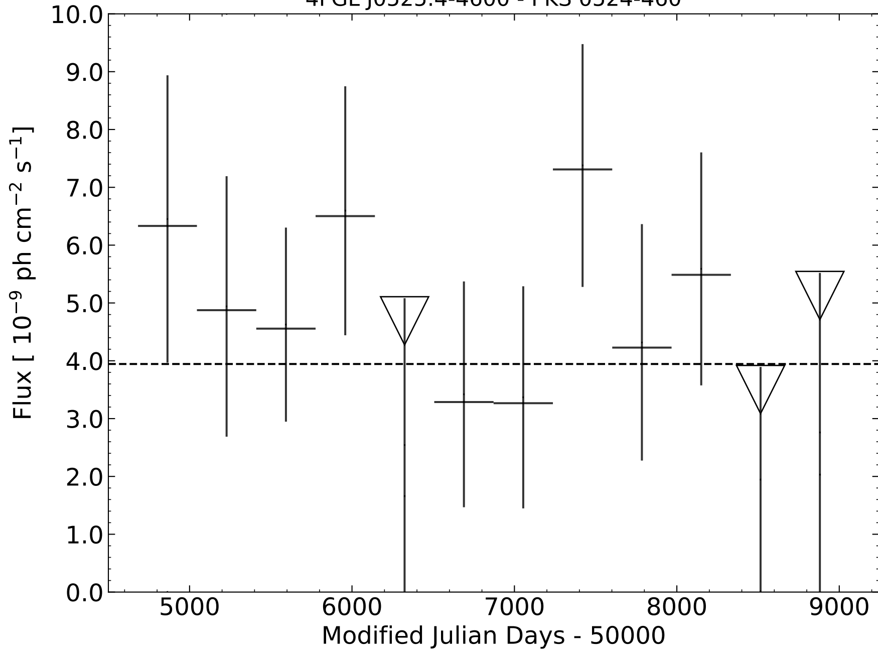
4FGL J0525.4-4600 - PKS 0524-460
