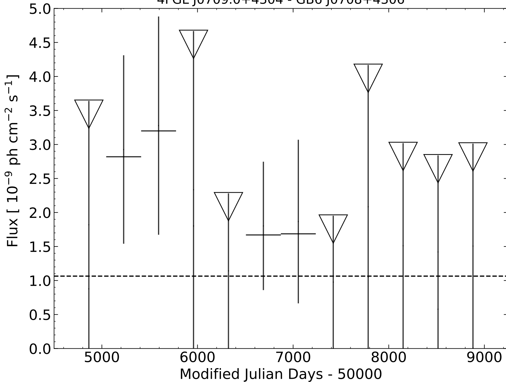
4FGL J0709.0+4304 - GB6 J0708+4306
