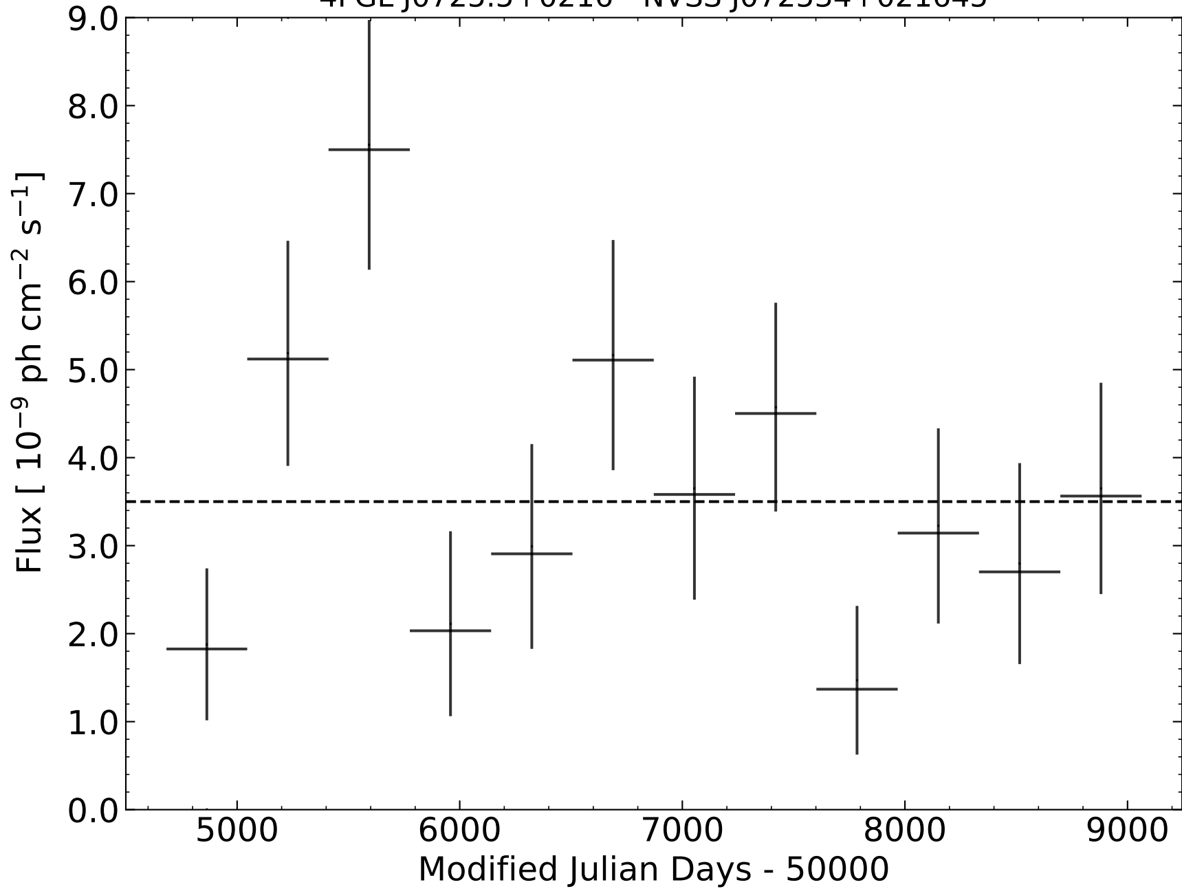
4FGL J0725.5+0216 - NVSS J072534+021645
