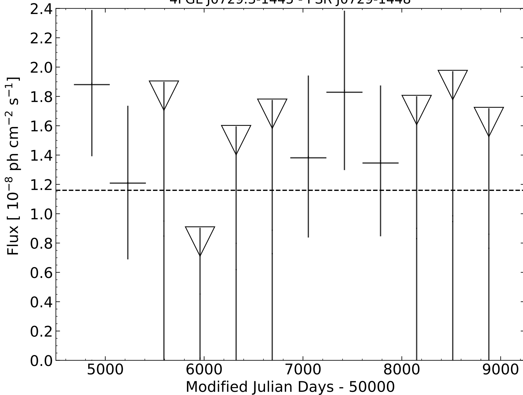
4FGL J0729.3-1445 - PSR J0729-1448
