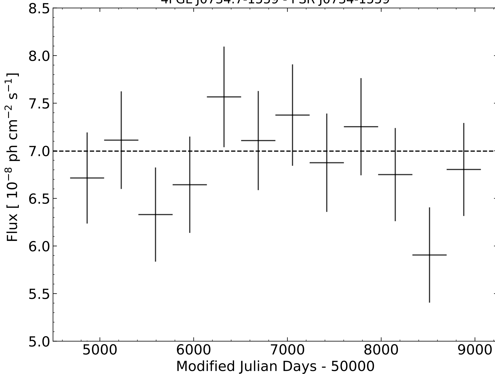
4FGL J0734.7-1559 - PSR J0734-1559
