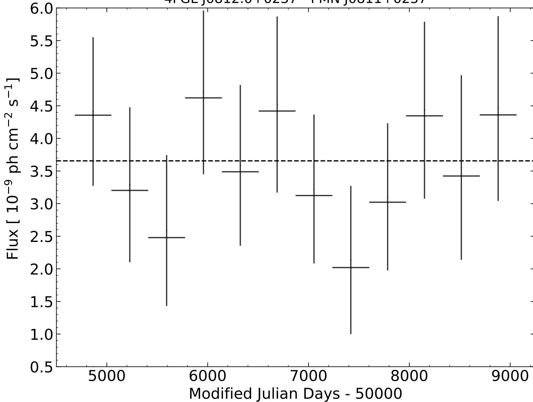
4FGL J0812.0+0237 - PMN J0811+0237
