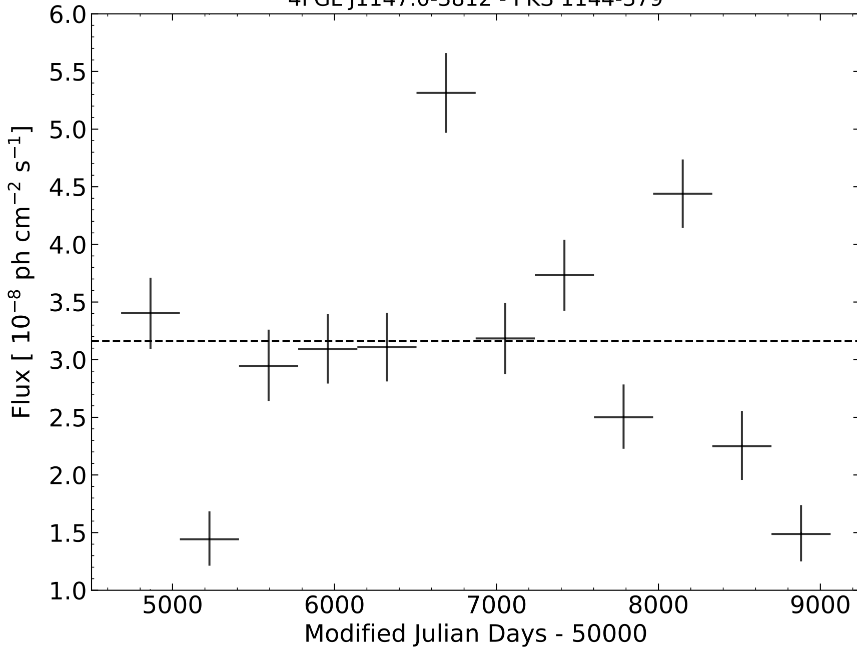
4FGL J1147.0-3812 - PKS 1144-379
