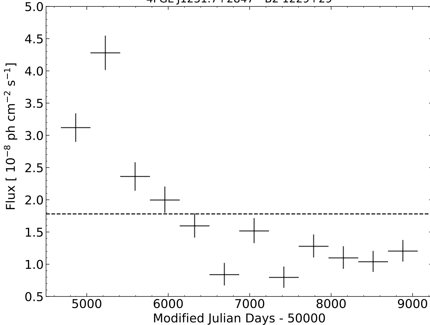
4FGL J1231.7+2847 - B2 1229+29
