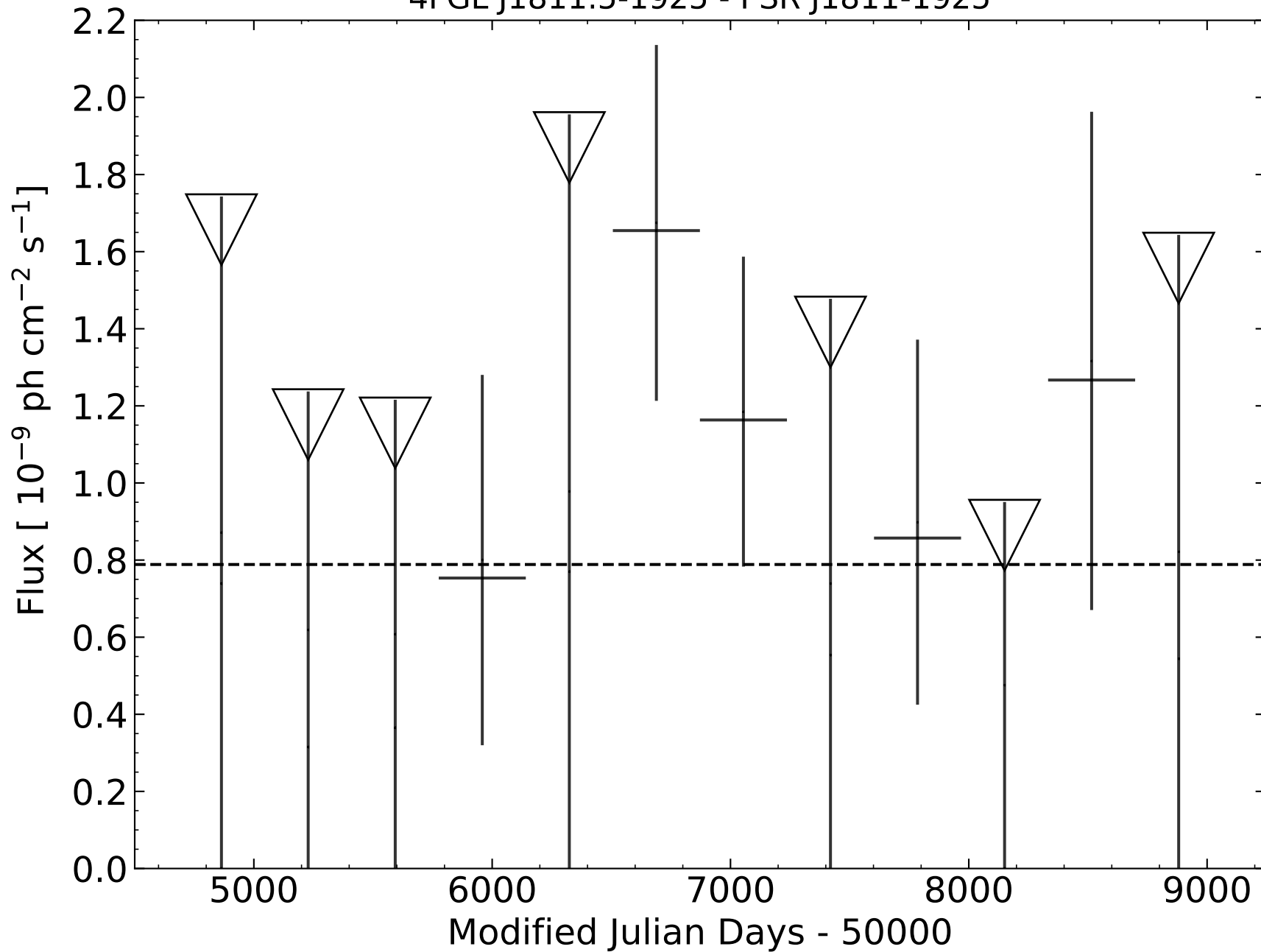
4FGL J1811.5-1925 - PSR J1811-1925
