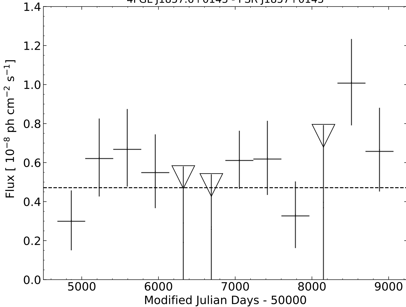
4FGL J1857.6+0143 - PSR J1857+0143
