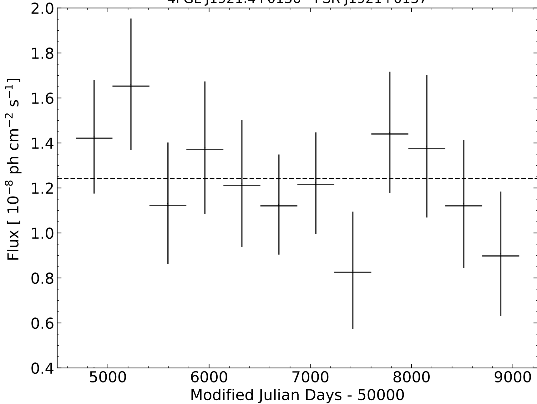
4FGL J1921.4+0136 - PSR J1921+0137
