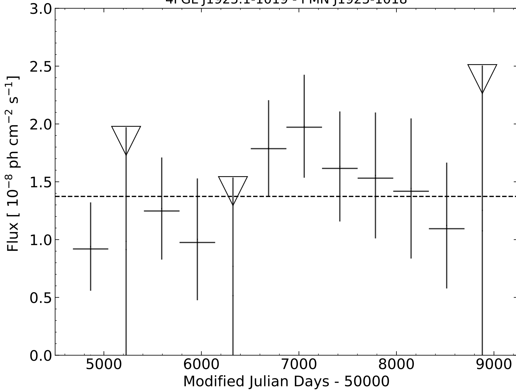
4FGL J1925.1-1019 - PMN J1925-1018
