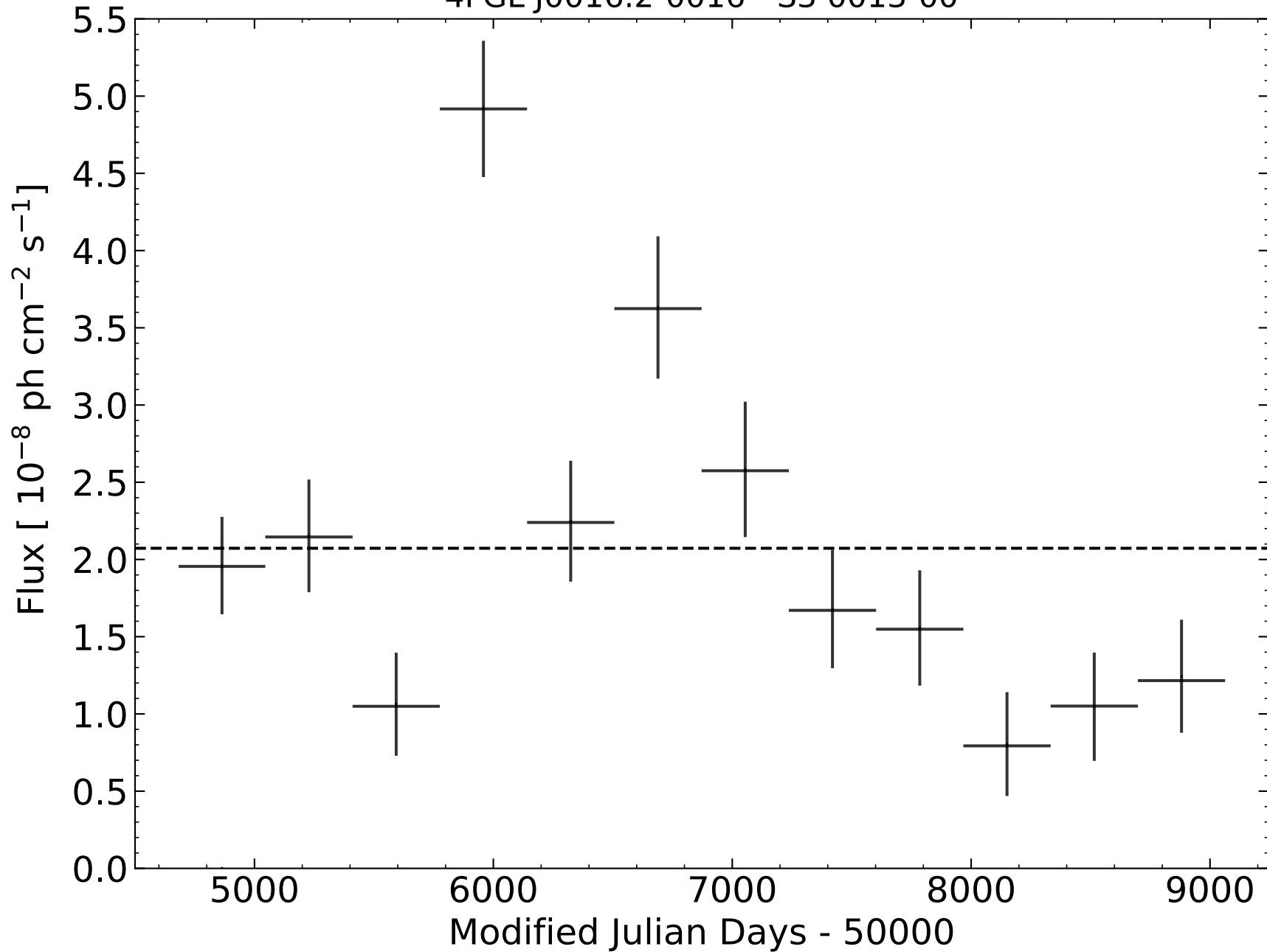
4FGL J0016.2-0016 - S3 0013-00
