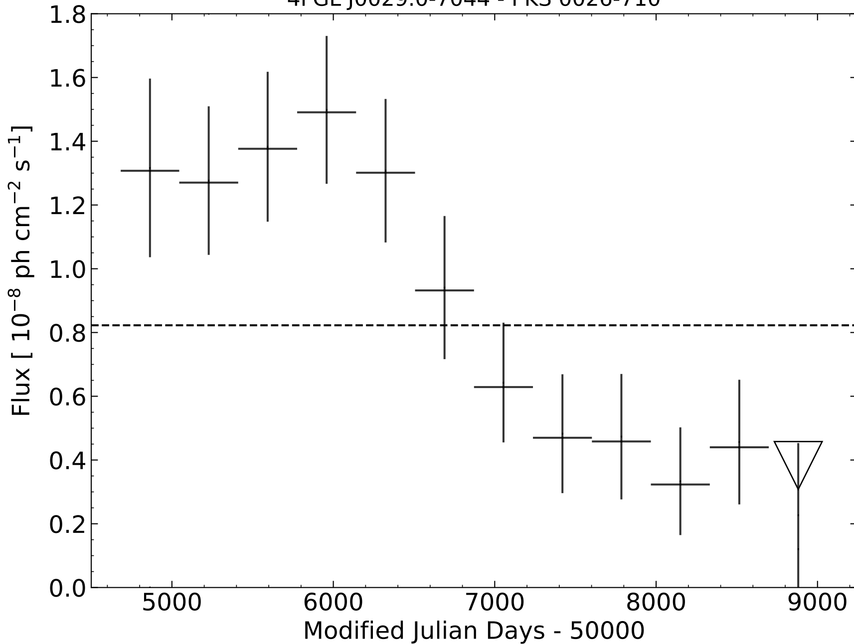
4FGL J0029.0-7044 - PKS 0026-710
