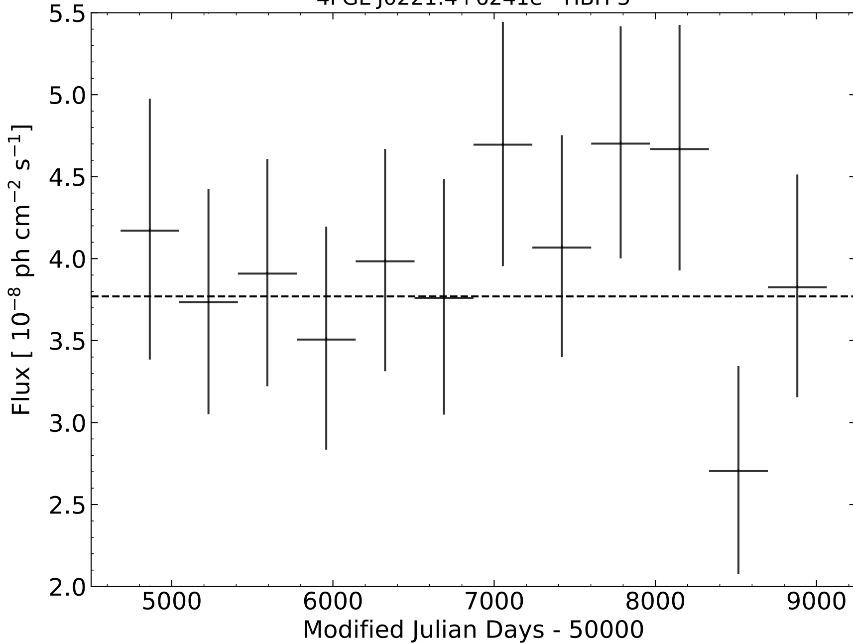
4FGL J0221.4+6241e - HBH 3
