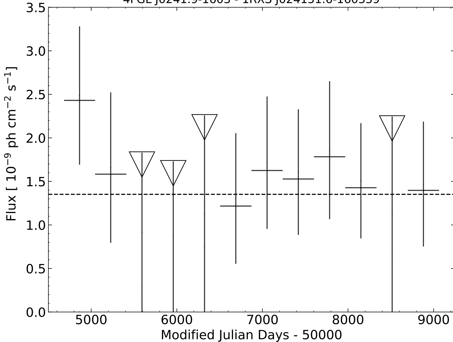
4FGL J0241.9-1603 - 1RXS J024151.6-160339
