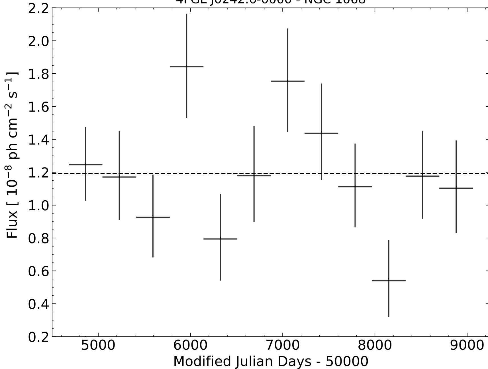
4FGL J0242.6-0000 - NGC 1068
