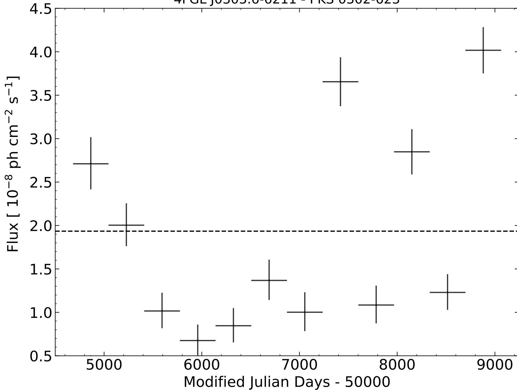
4FGL J0303.6-6211 - PKS 0302-623
