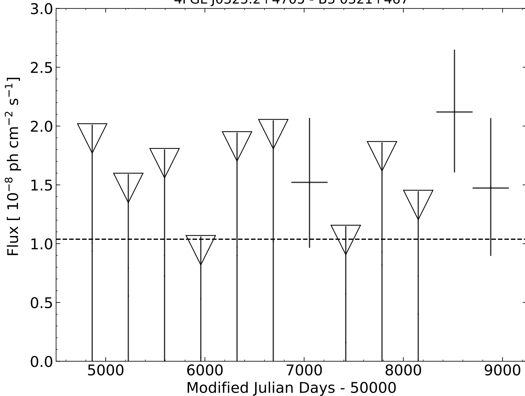
4FGL J0325.2+4705 - B3 0321+467
