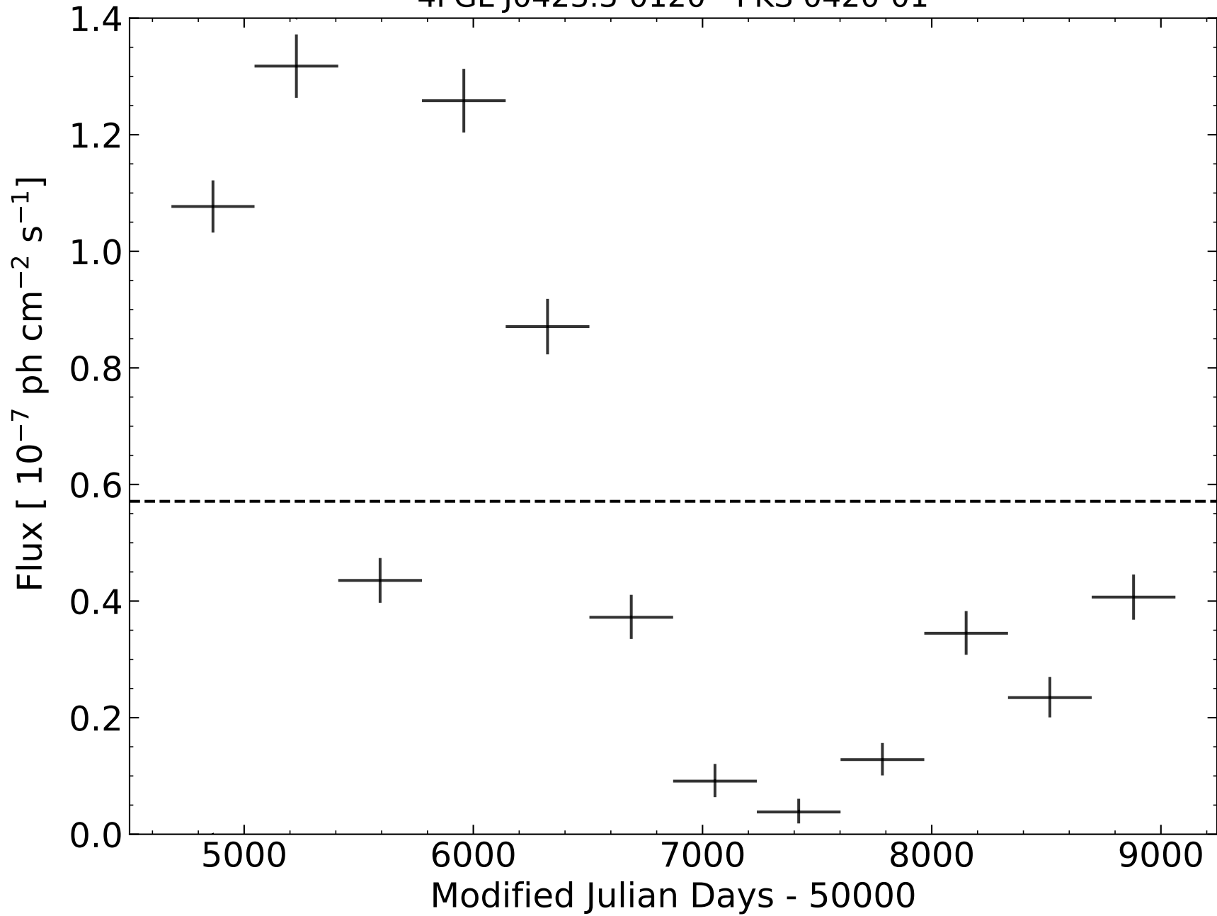
4FGL J0423.3-0120 - PKS 0420-01
