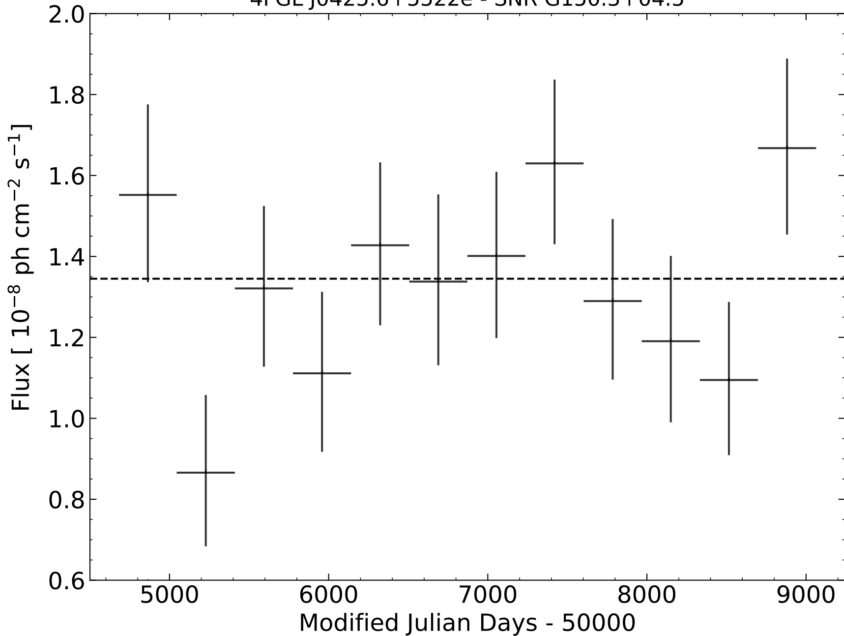
4FGL J0425.6+5522e - SNR G150.3+04.5
