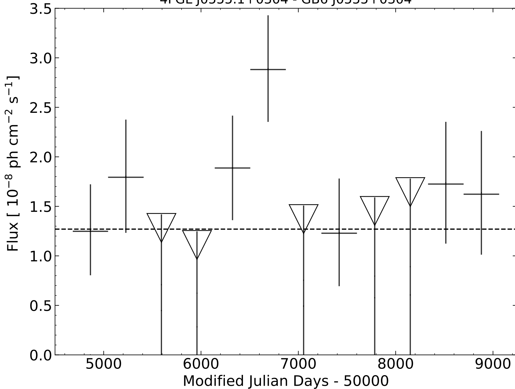
4FGL J0555.1+0304 - GB6 J0555+0304
