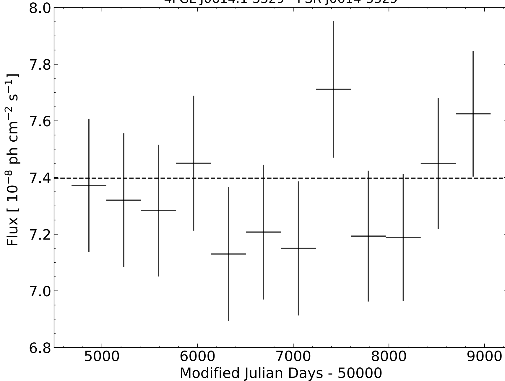
4FGL J0614.1-3329 - PSR J0614-3329
