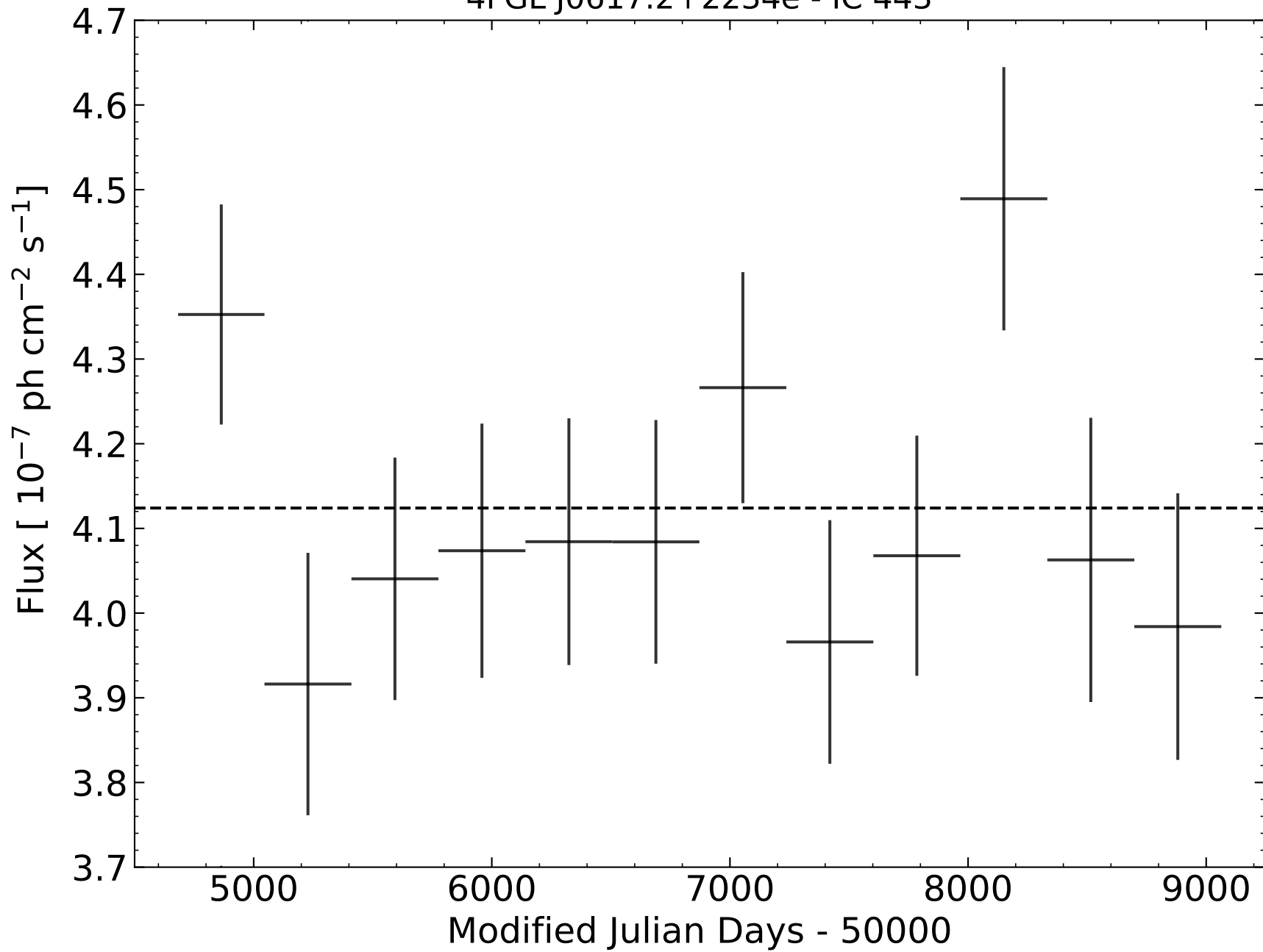
4FGL J0617.2+2234e - IC 443
