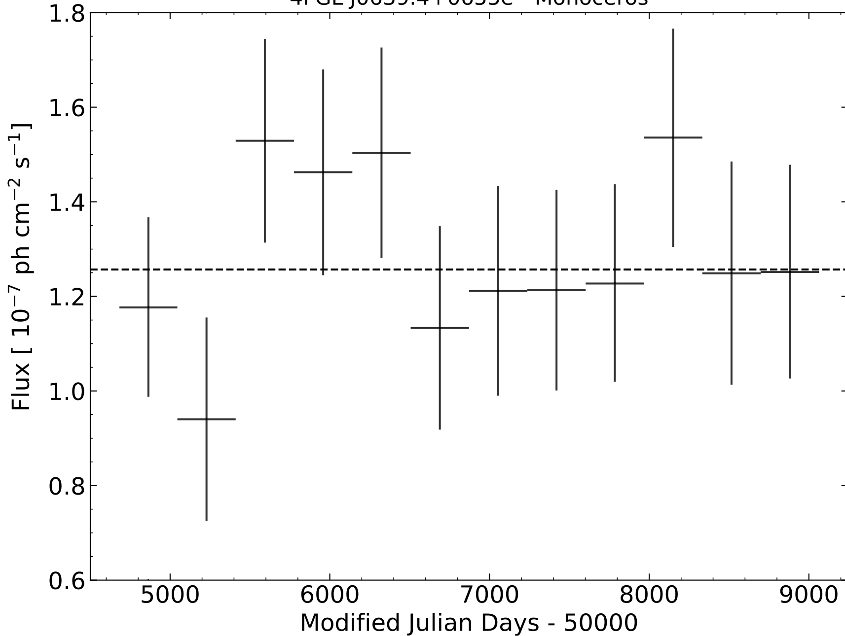
4FGL J0639.4+0655e - Monoceros
