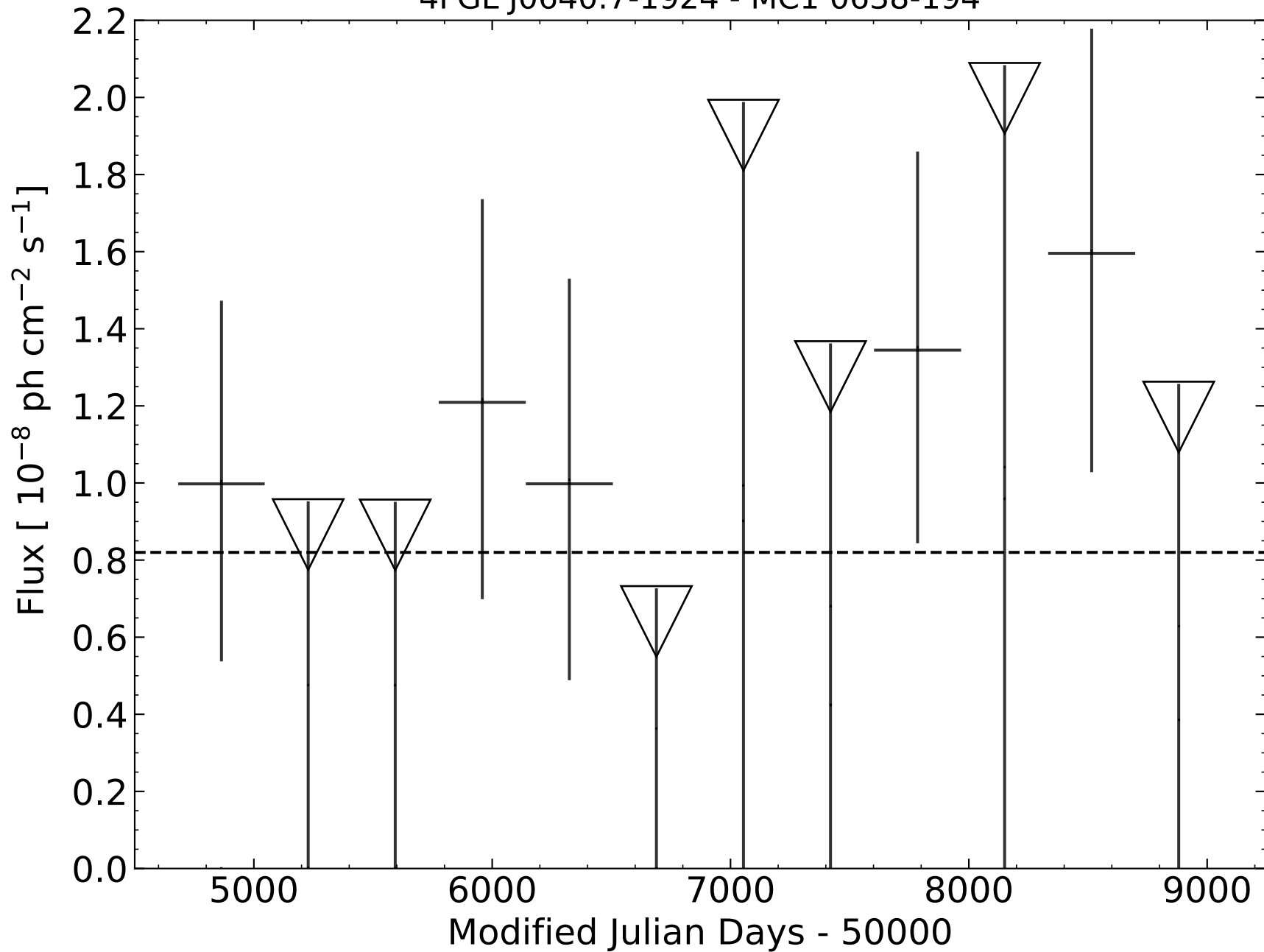
4FGL J0640.7-1924 - MC1 0638-194
