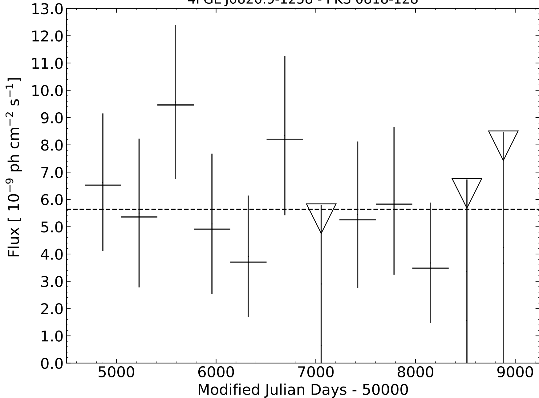
4FGL J0820.9-1258 - PKS 0818-128
