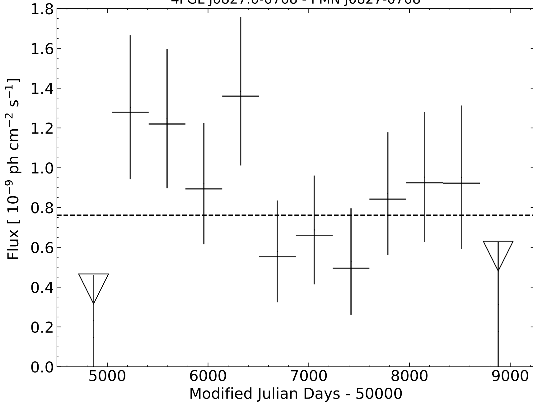
4FGL J0827.0-0708 - PMN J0827-0708
