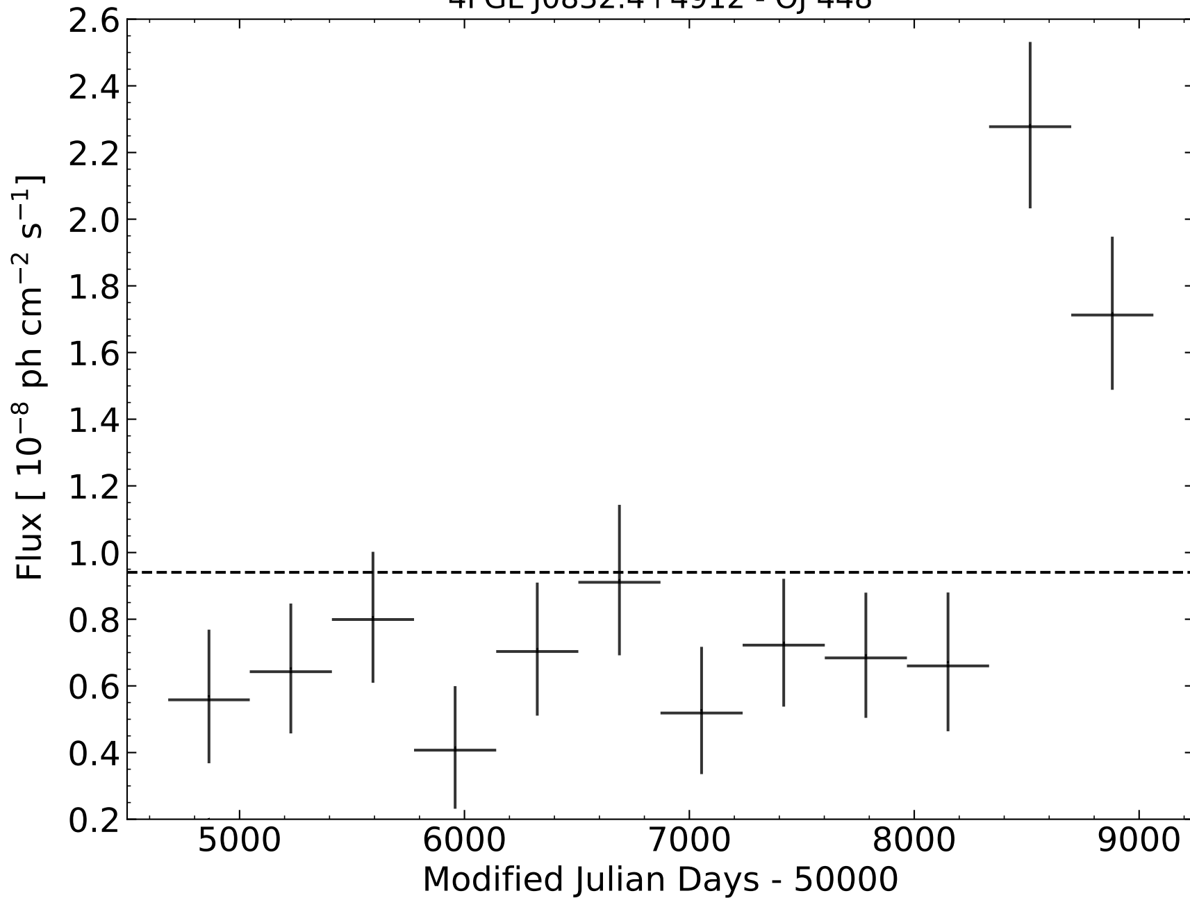
4FGL J0832.4+4912 - OJ 448
