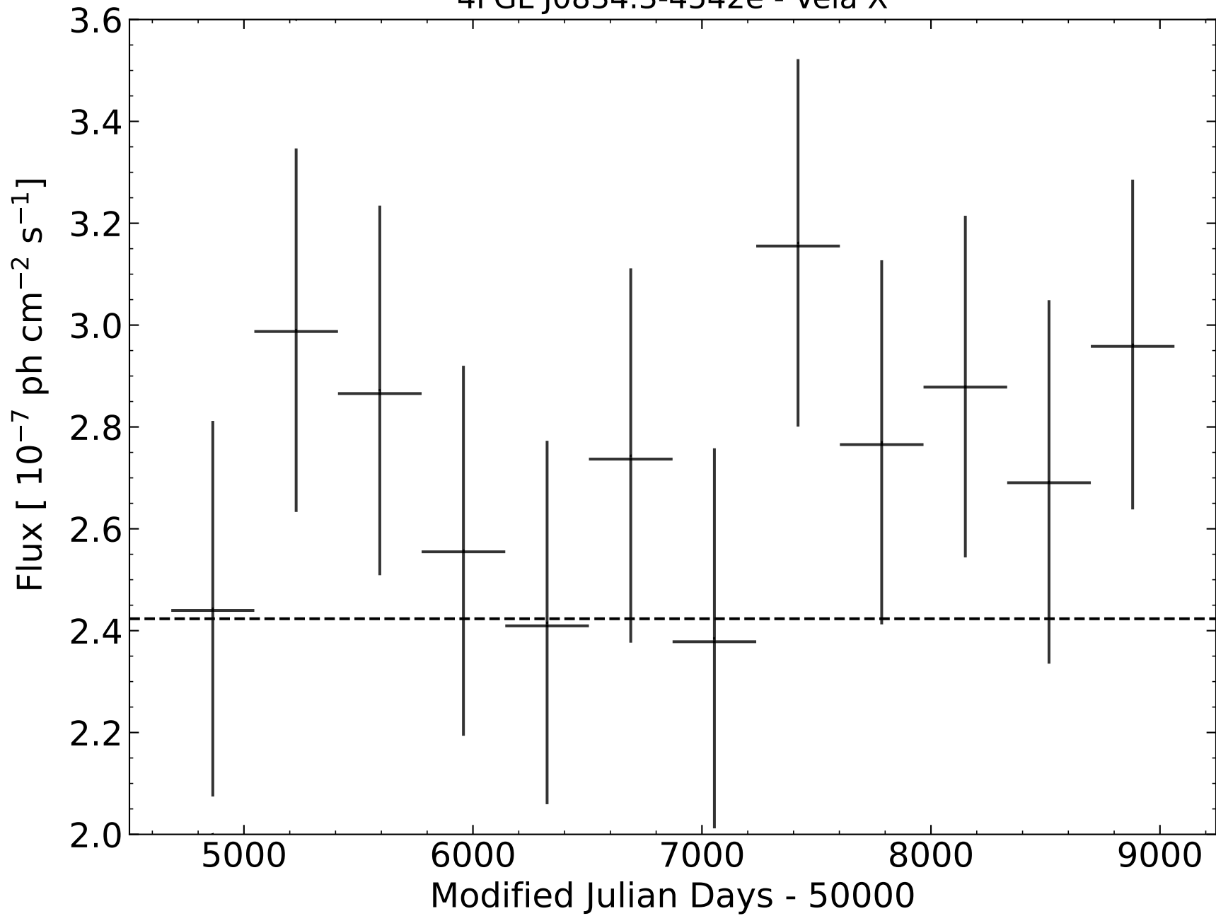
4FGL J0834.3-4542e - Vela X
