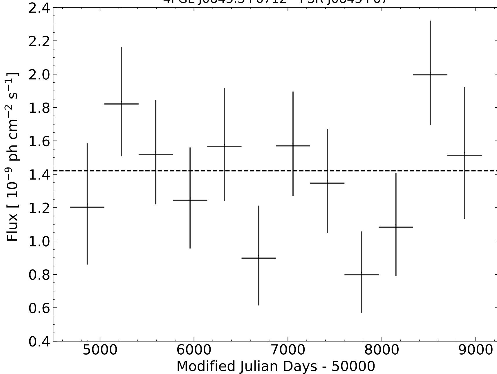
4FGL J0843.3+6712 - PSR J0843+67
