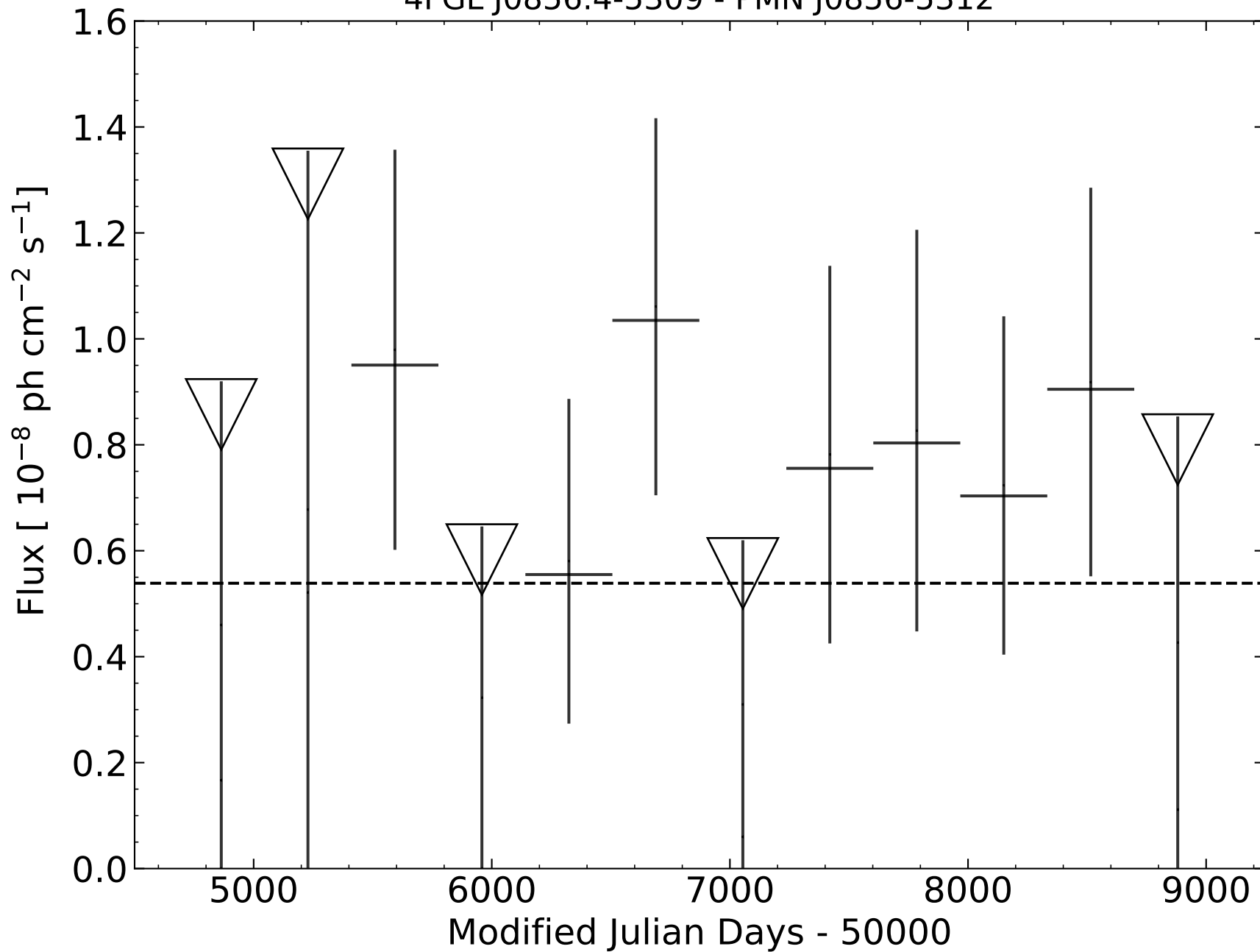
4FGL J0856.4-5309 - PMN J0856-5312
