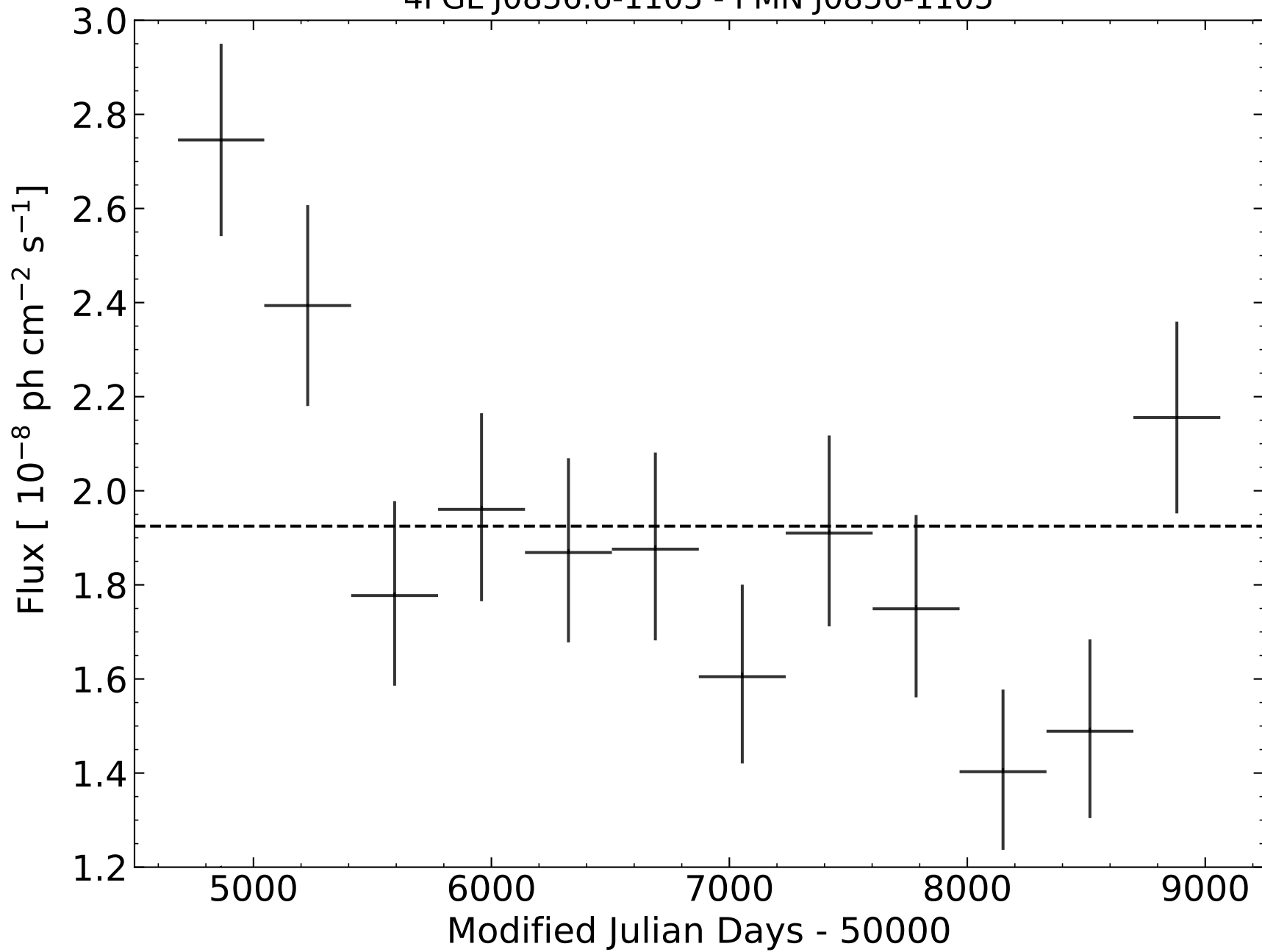
4FGL J0856.6-1105 - PMN J0856-1105
