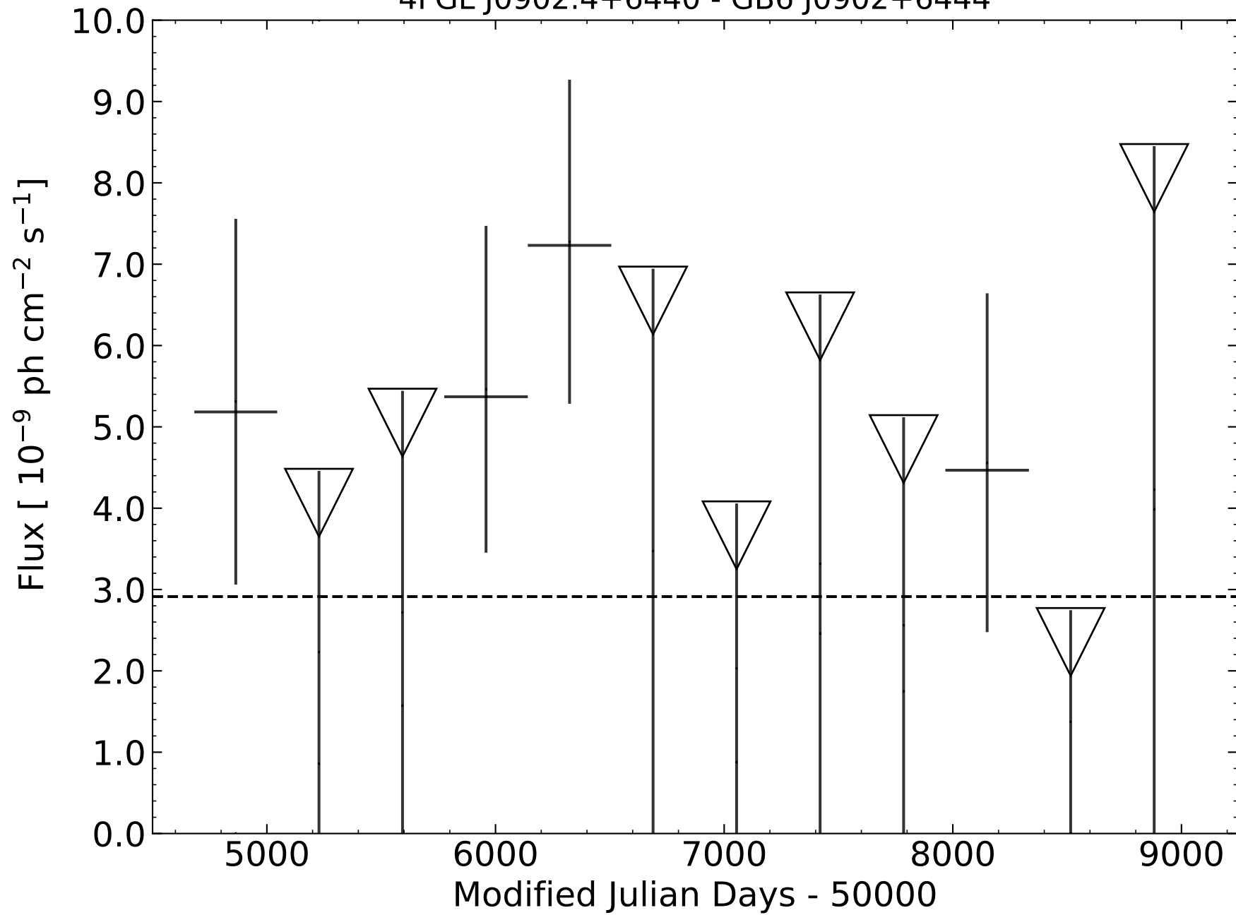
4FGL J0902.4+6440 - GB6 J0902+6444
