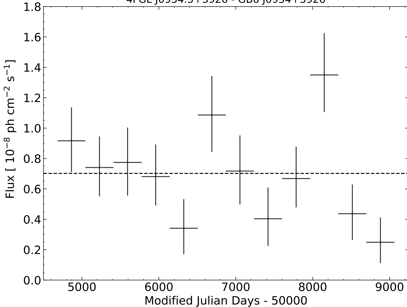
4FGL J0934.3+3926 - GB6 J0934+3926
