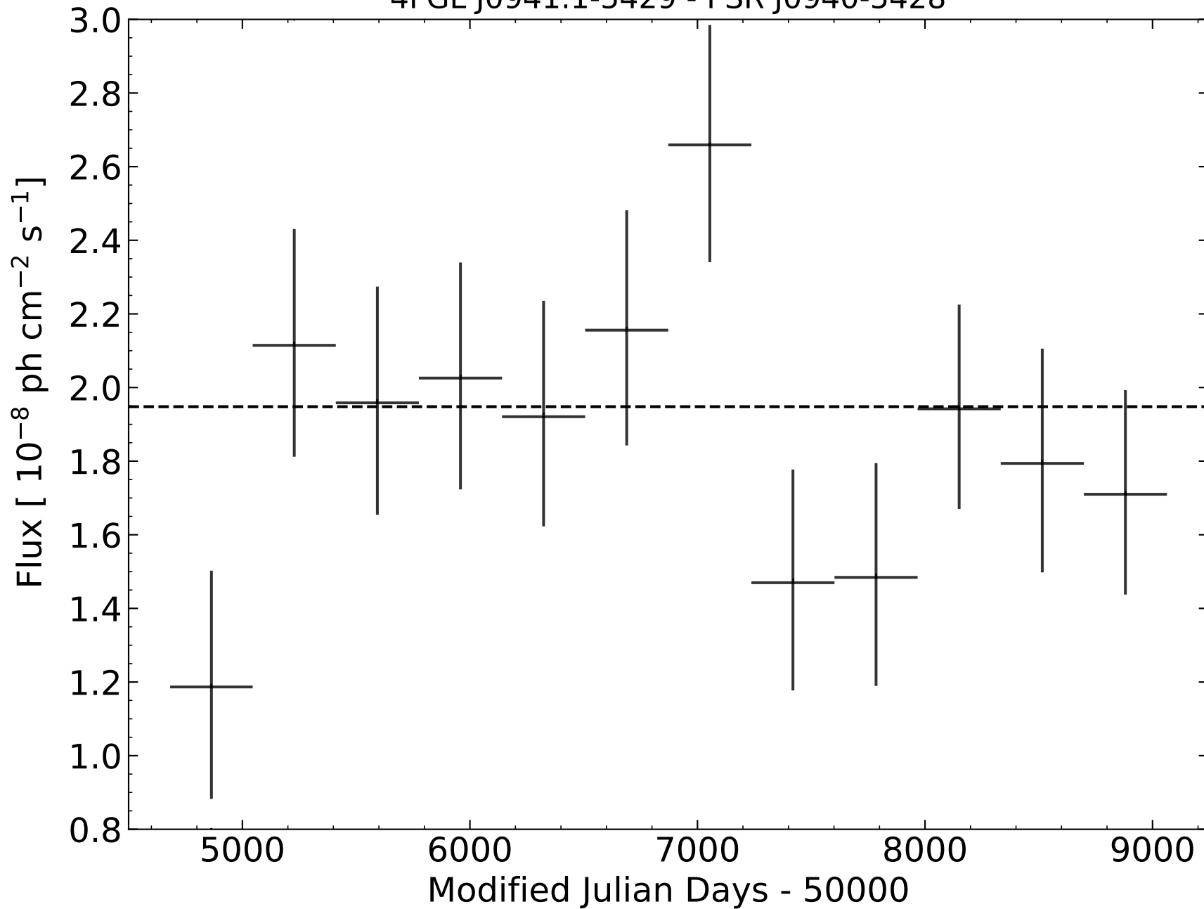
4FGL J0941.1-5429 - PSR J0940-5428
