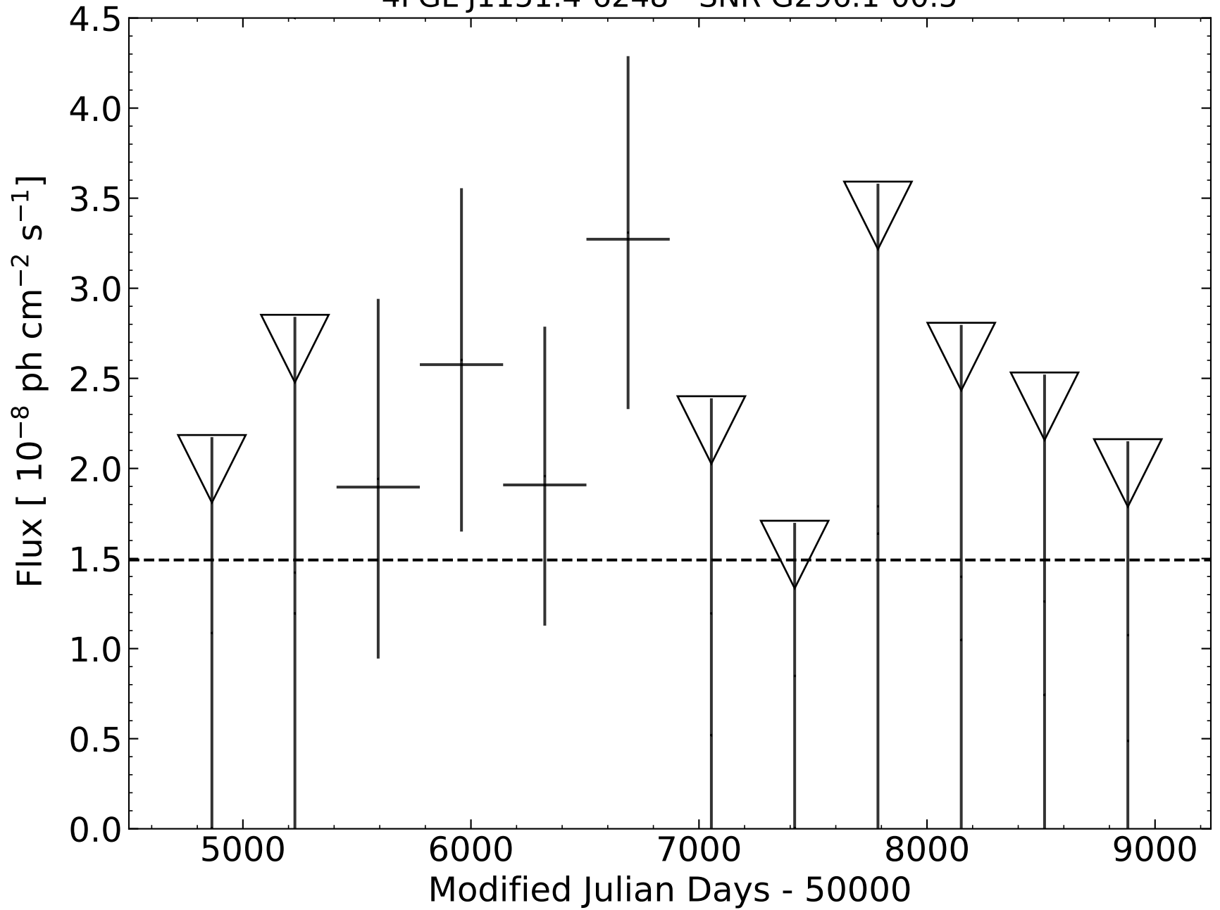
4FGL J1151.4-6248 - SNR G296.1-00.5
