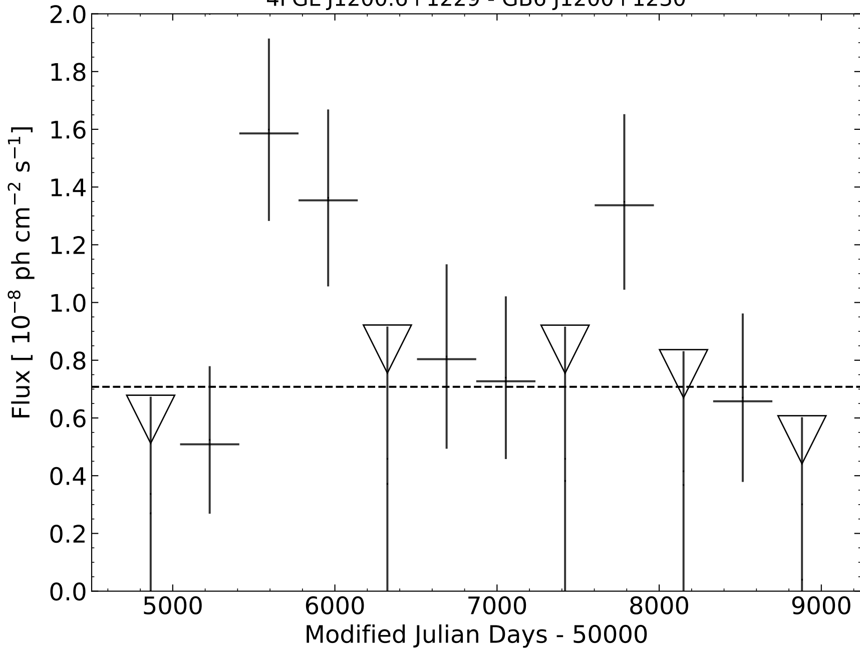
4FGL J1200.6+1229 - GB6 J1200+1230
