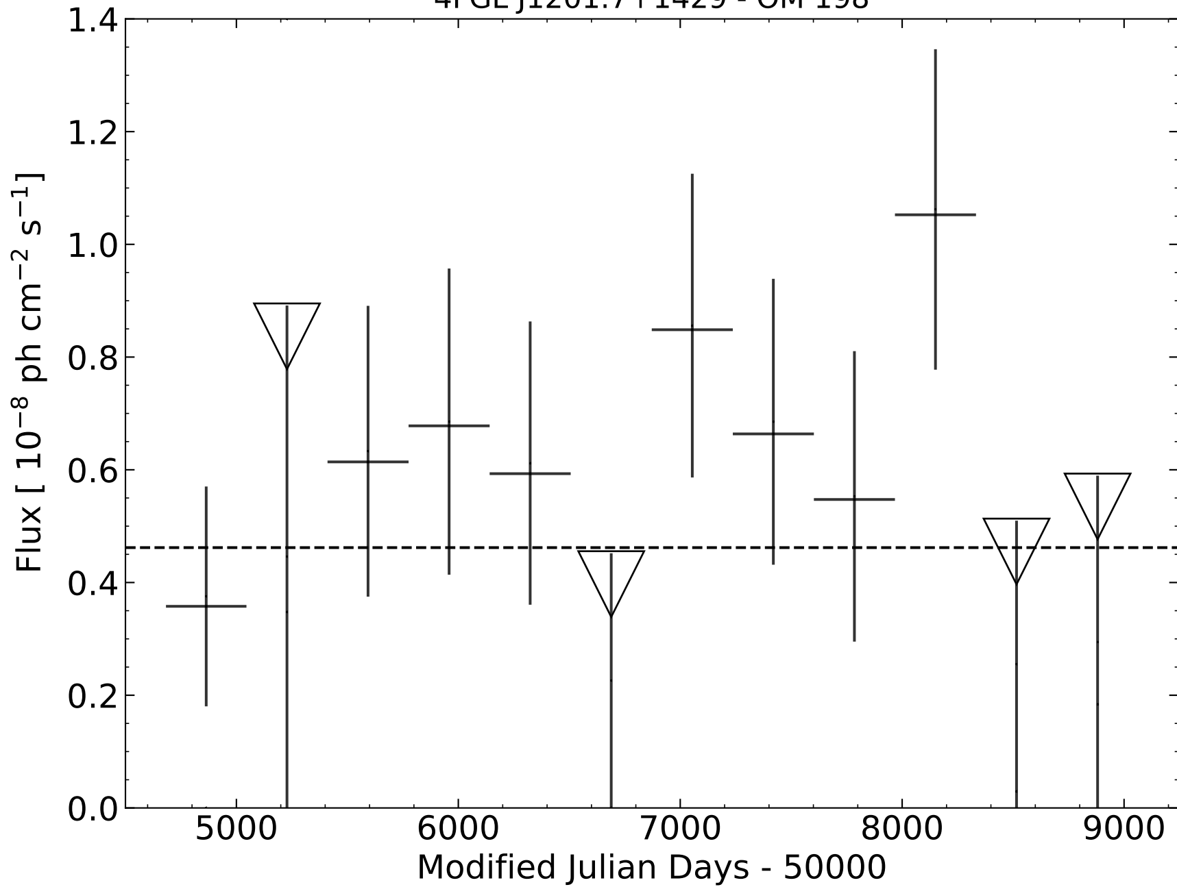
4FGL J1201.7+1429 - OM 198
