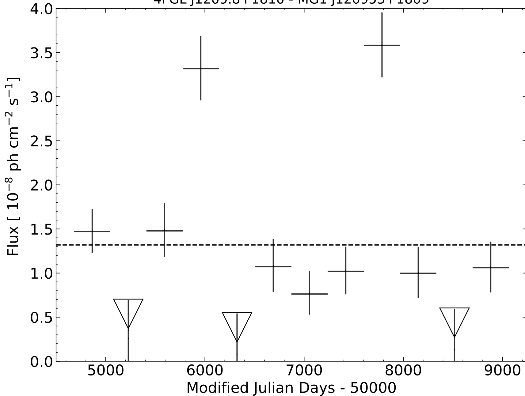
4FGL J1209.8+1810 - MG1 J120953+1809
