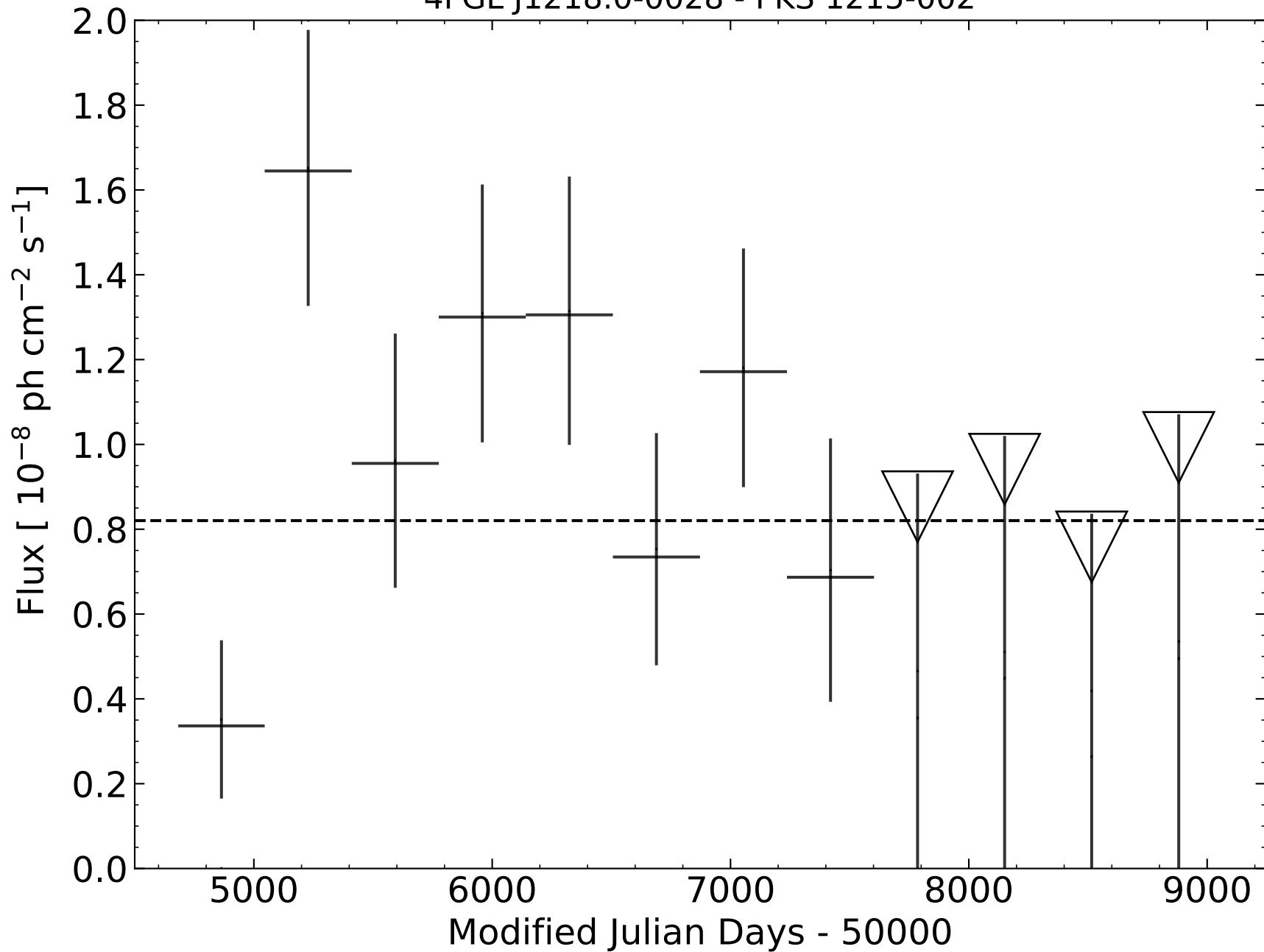
4FGL J1218.0-0028 - PKS 1215-002
