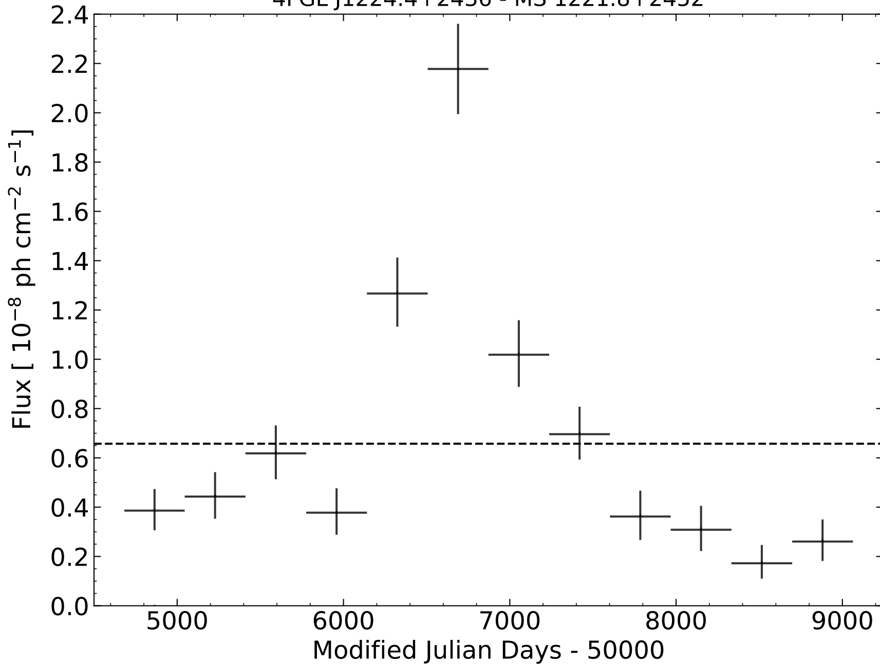
4FGL J1224.4+2436 - MS 1221.8+2452
