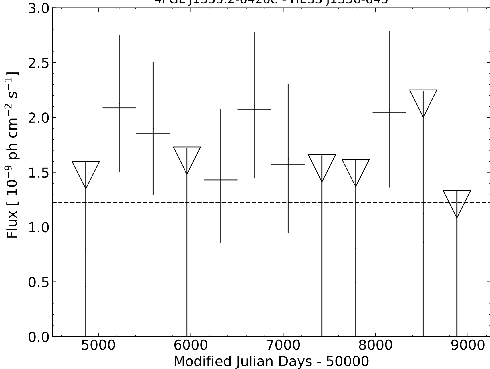
4FGL J1355.2-6420e - HESS J1356-645
